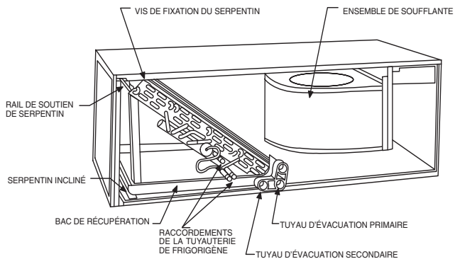
Fig. 5 - Conversion en application horizontale droite Avec serpentin incliné (FB4C seulement)
