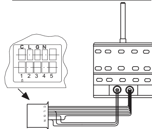
Fig. 18 - Sélection de vitesse du moteur (FB4C seulement)
