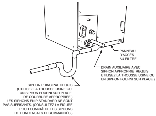
Fig. 21 - Siphon de condensat et appareil
