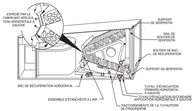
Fig. 3 - Serpentin en A pour une application horizontale gauche (appareil FB4C configuré en usine seulement)
