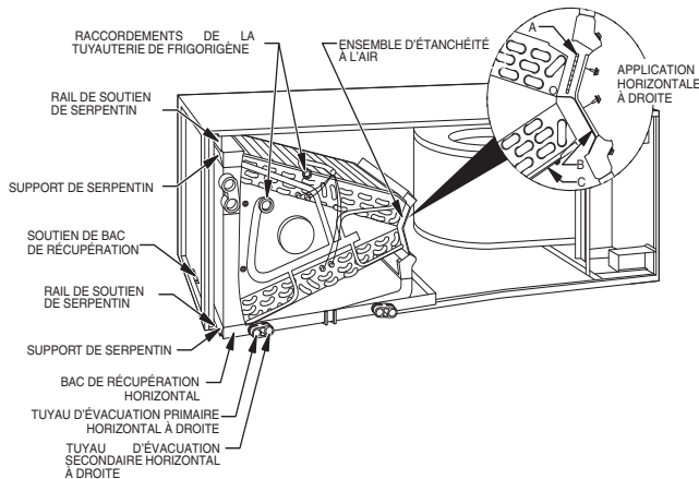
Fig. 6 - Conversion en application horizontale droite Avec serpentin en A (FB4C seulement)
