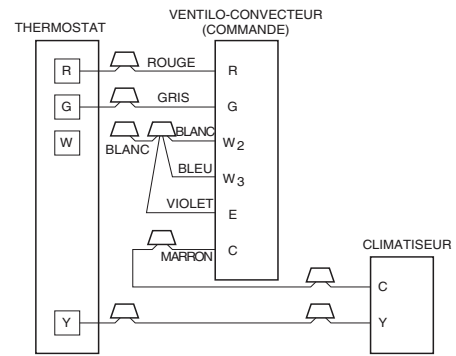
Fig. 10 - Agencement du câblage – Climatiseur (refroidissement seulement)
