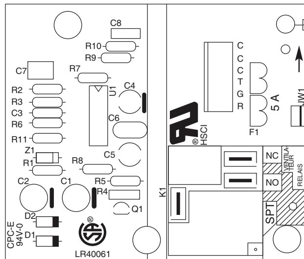
Fig. 9 - Carte de circuit imprimé du ventilateur-convecteur FY5B
