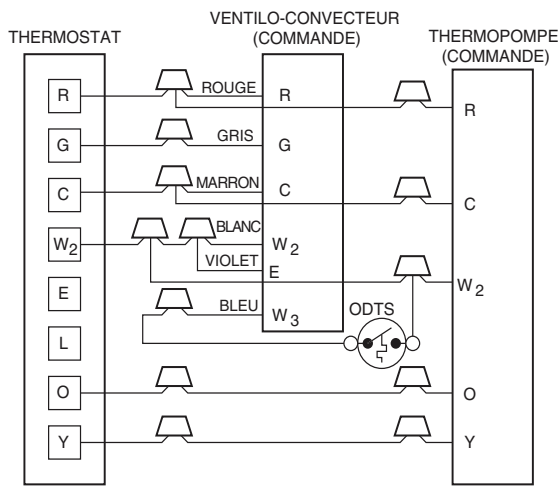
Fig. 13 - Agencement du câblage – Thermopompe (refroidissement et chauffage 2 étages avec 1 thermostat extérieur)
