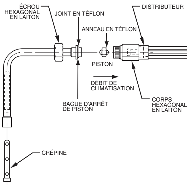
Fig. 19 - Dispositif de commande de débit de frigorigène
