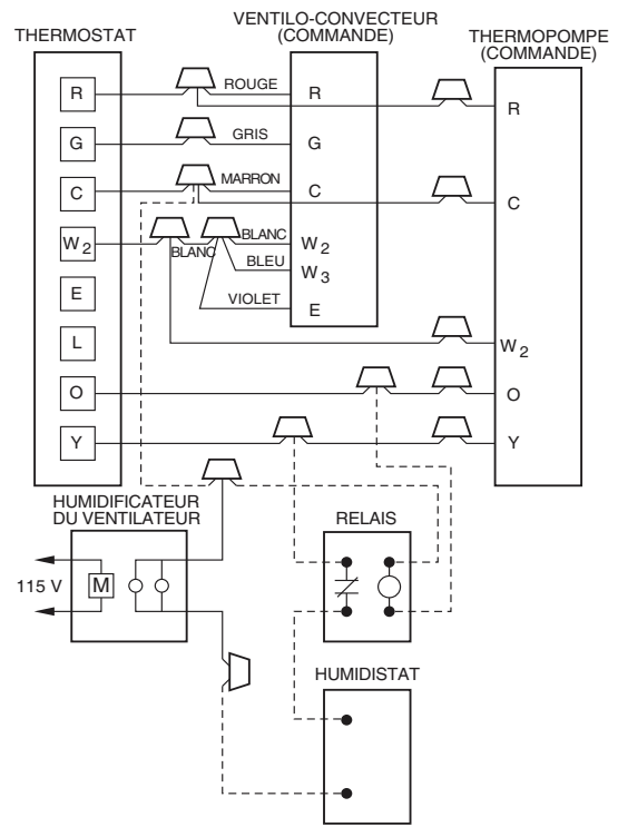
Fig. 24 - Disposition du câblage de l'humidificateur vers la thermopompe
