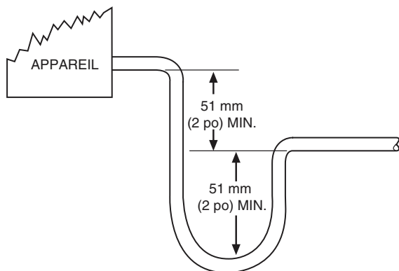
Fig. 20 - Siphon de condensat recommandé
