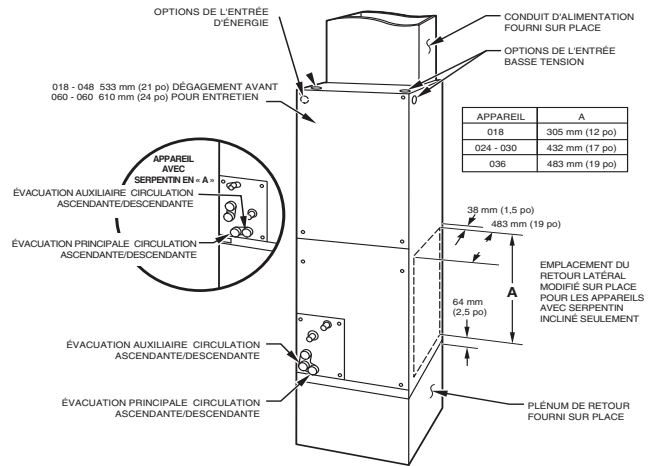
Fig. 1 - Appareil avec serpentin incliné dans une configuration à tirage ascendant
