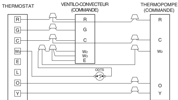
Fig. 14 - Agencement du câblage – Thermopompe (refroidissement et chauffage 2 étages avec deux thermostats extérieurs)
