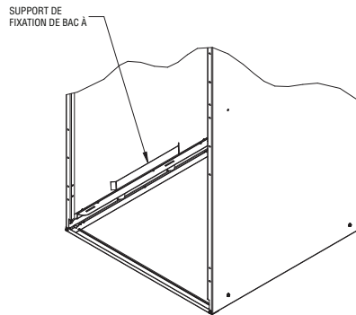
Fig. 7 - Support de fixation du bac à condensats
