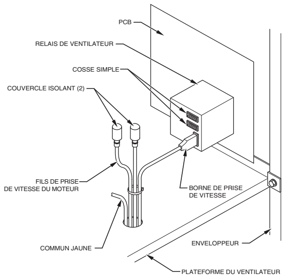
Fig. 17 - Relai et borne de prise de vitesse pour ventilo-convecteurs FY5B
