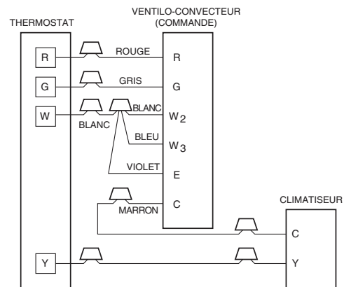
Fig. 10 - Agencement du câblage – Climatiseur (refroidissement seulement)
